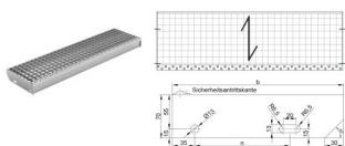
Feuerverzinkte Gitterrost-Treppenstufe, Maschenweite 3 x 3 cm, mit Sicherheits-Antrittskante
